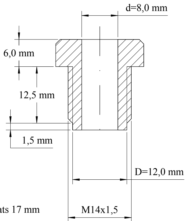
Längsschnitt 2:1 cross-cut view
